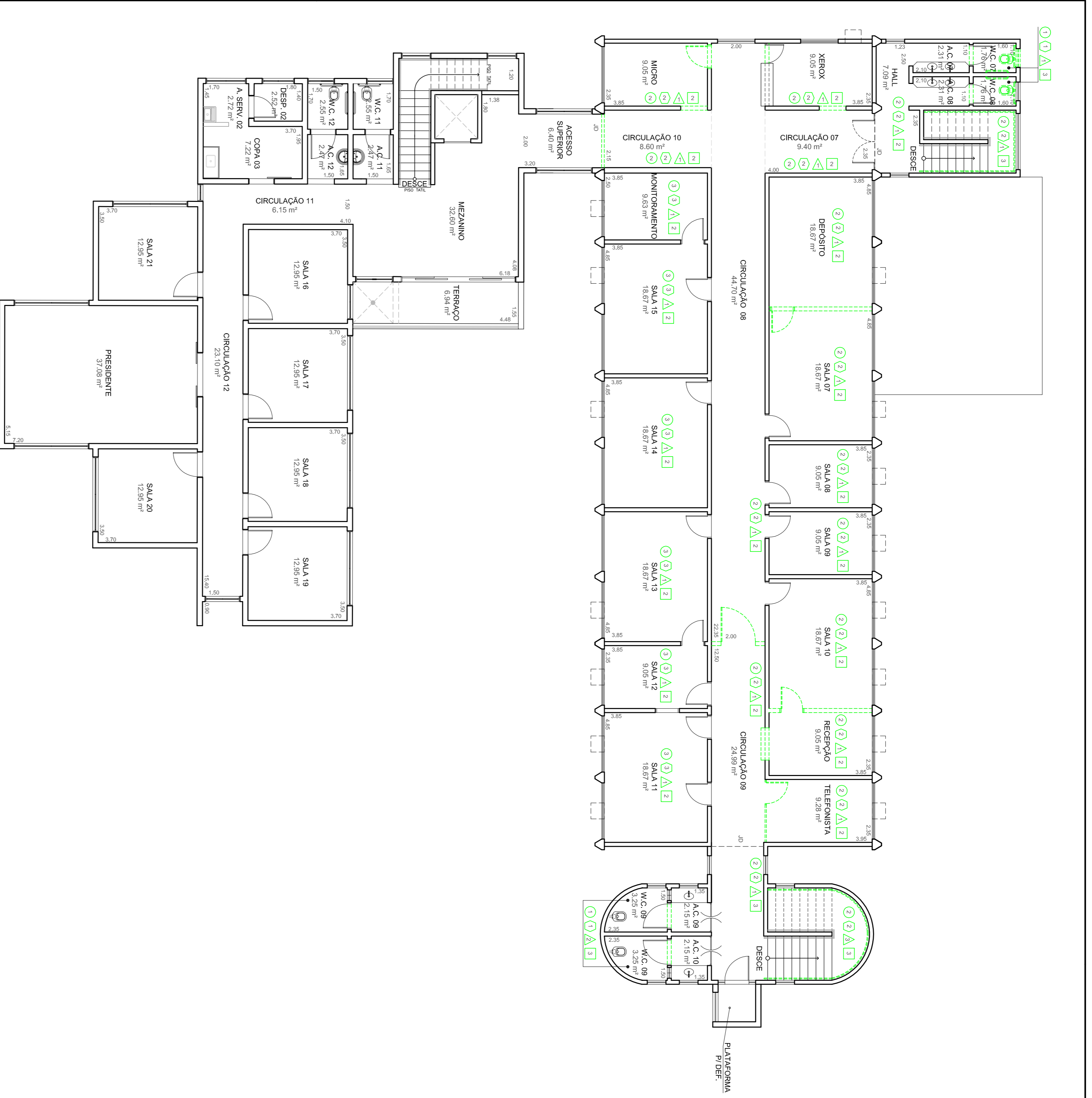
PAVIMENTO SUPERIOR DEMOLIR/ RETIRAR ESC.: 1:100
